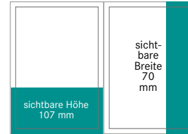
1/3 Seite quer 1/3 Seite hoch Breite 216 mm Breite 73 mm Höhe 112 mm Höhe 307 mm
